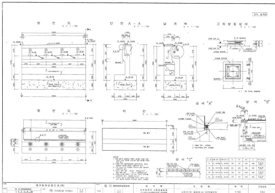
<그림 1.2.1> 주요도면(계속)
